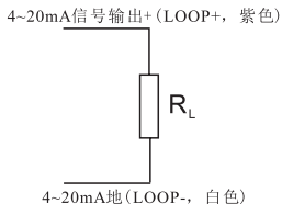
(图6-6) 4~20mA信号输出外部接线图
