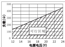
(图6-7) 负载与电源电压关系图
